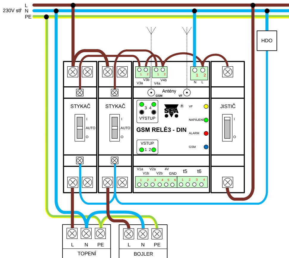
Drátové zapojení
